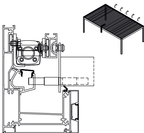
Secțiune transversală a șinei de ghidare longitudinale
