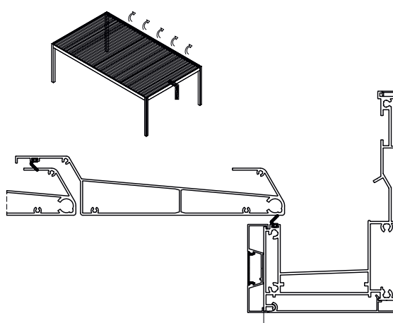
Secțiune transversală a șinei de ghidare
